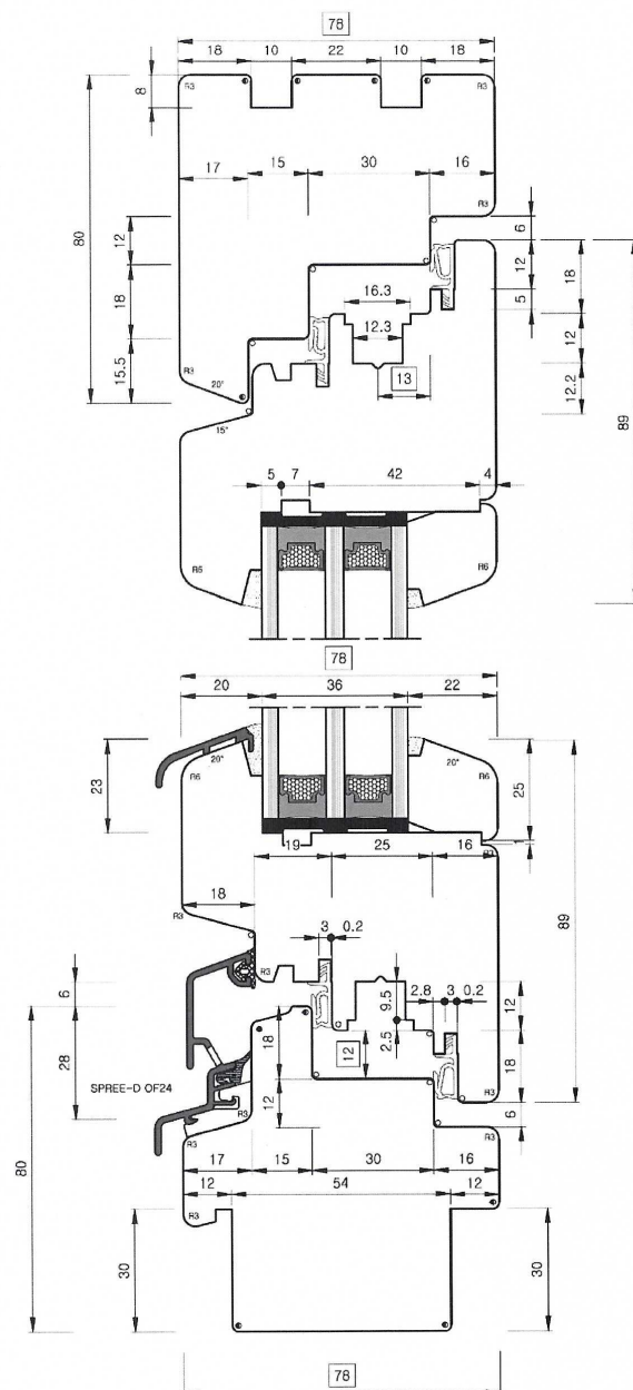
Obr. č. 1 Řez horním a dolním dílem
