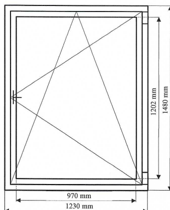
Obr. č. 2 Znáznornění rozměrů vzorku pro výpočet A_g , A_f a I_g
